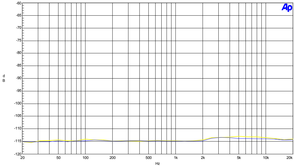
LPA-2a + SIA-5.V2 THD+N über die Frequenz bei 2x 500 mW an 100 Ω
