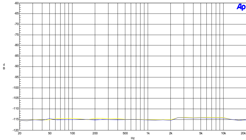
LPA-2a + SIA-5.V2 THD+N über die Frequenz bei 2x 10 mW an 600 Ω
