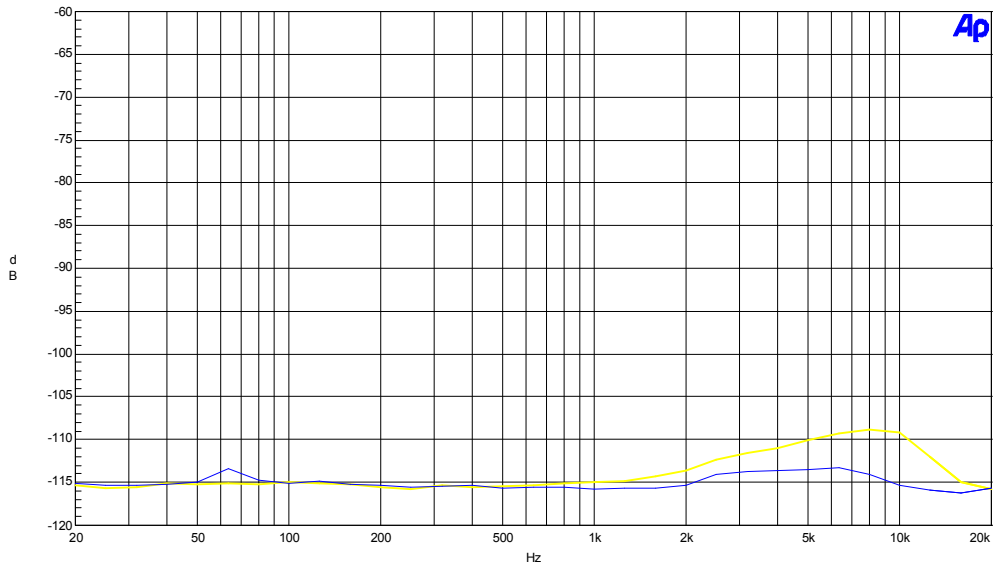
LPA-2a + SIA-5.V2 THD+N über die Frequenz bei 2x 250 mW an 32 Ω
