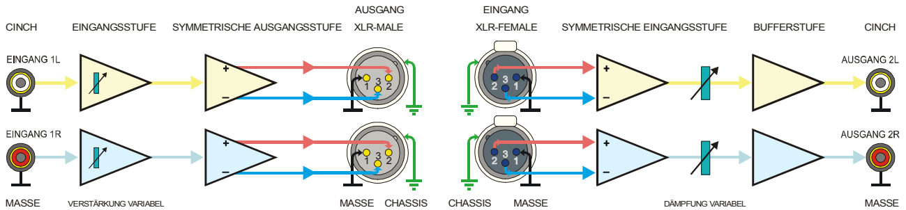
Blockschaltbild SAM-2C/2-2 1 Stereo-Symmetriermodule und 1 Stereo-Differenzverstärkermodul
