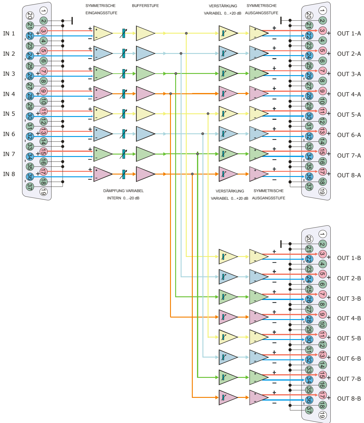
vollsymmetrischer Anpassverstärker SAM-3B.V2/16v8
