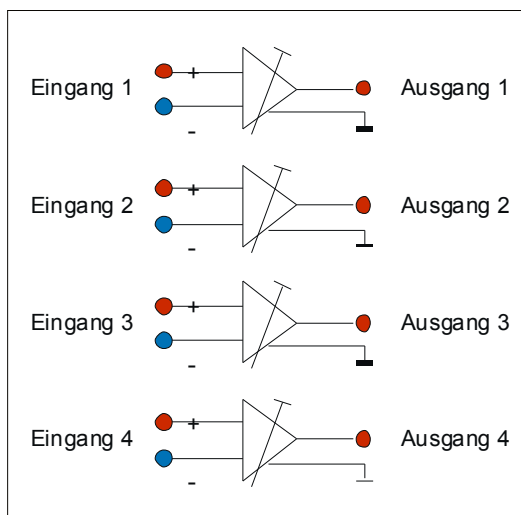
vereinfachtes Blockschaltbild
