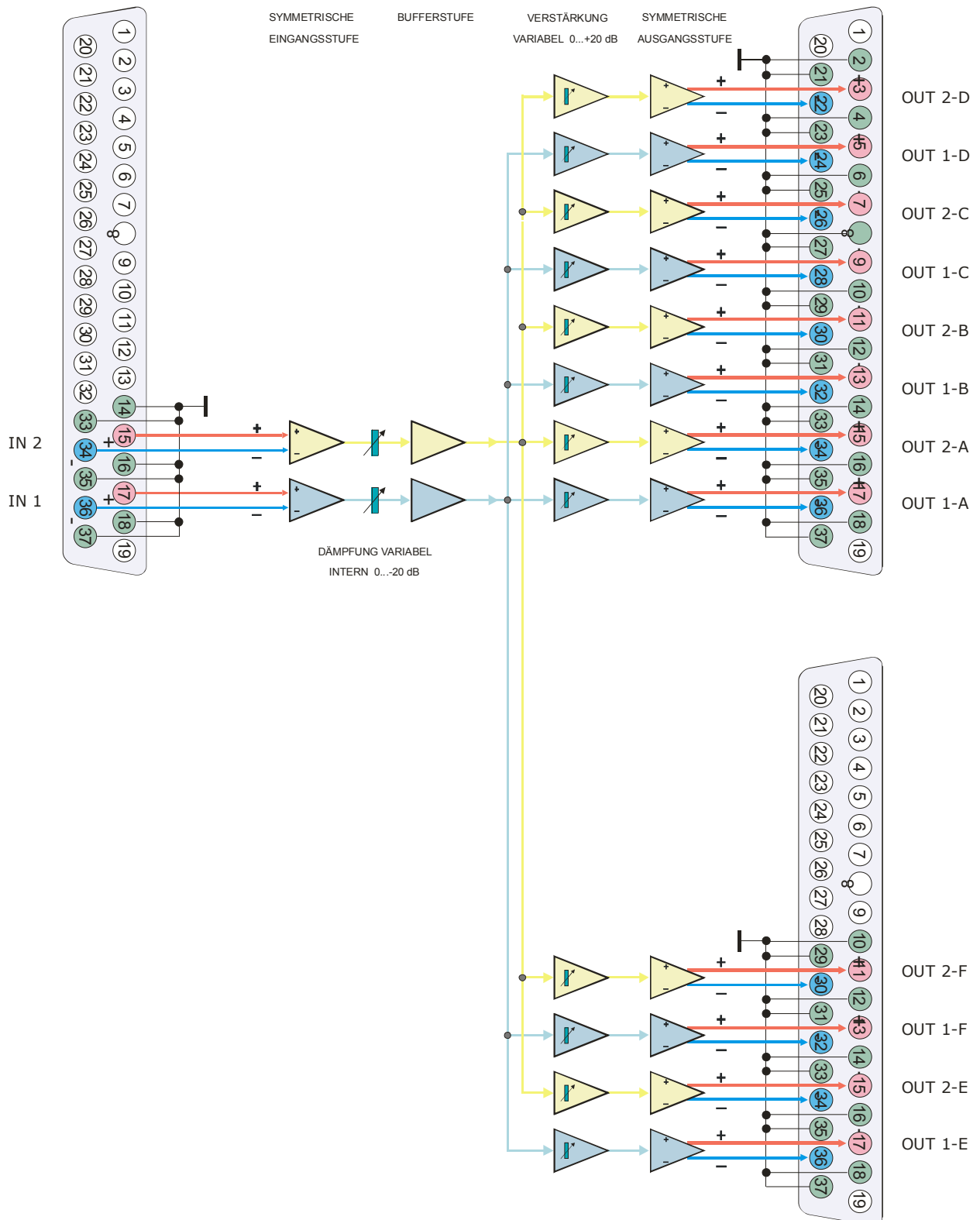
vollsymmetrischer Verteilverstärker SAM-3B.V2/12v2
