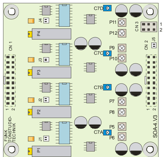
Lage der Jumper und Steckverbinder
