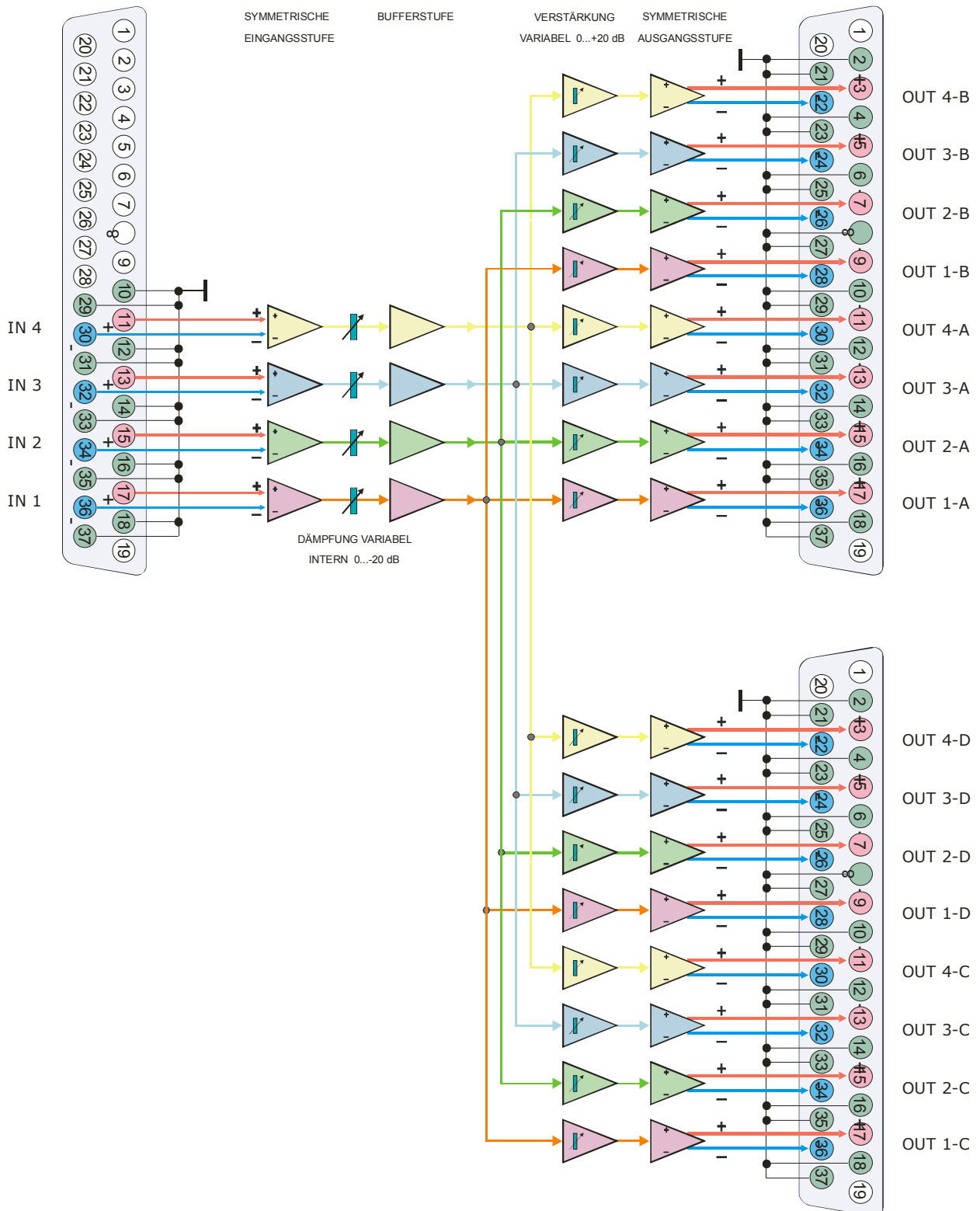
vollsymmetrischer Verteilverstärker SAM-3B.V2/16v4
