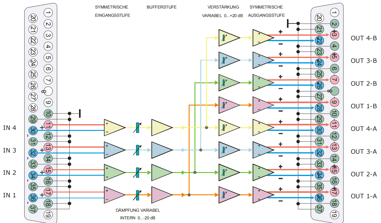
vollsymmetrischer Verteilverstärker SAM-3B.V2/8v4
