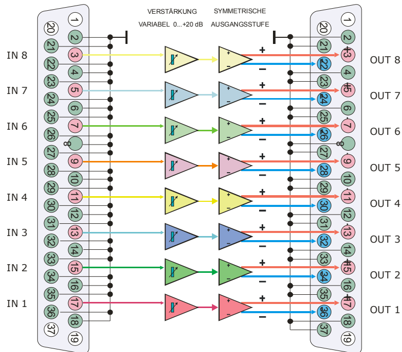
Symmetrier- und Differenzverstärker SAM-3B.V2/8-8
