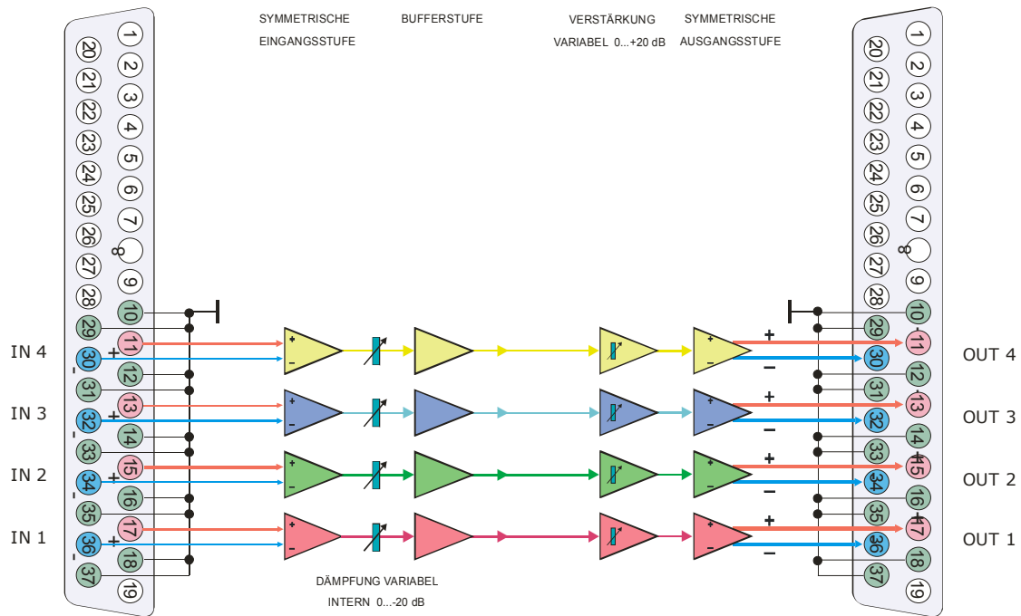
vollsymmetrischer Anpassverstärker SAM-3B.V2/4SVS4
