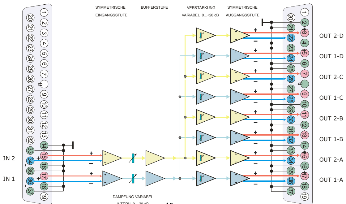
vollsymmetrischer Verteilverstärker SAM-3B.V2/8v2
