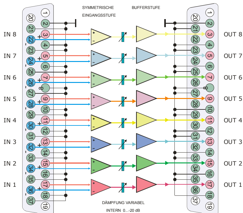
Differenzverstärker SAM-3B.V2/0-8
