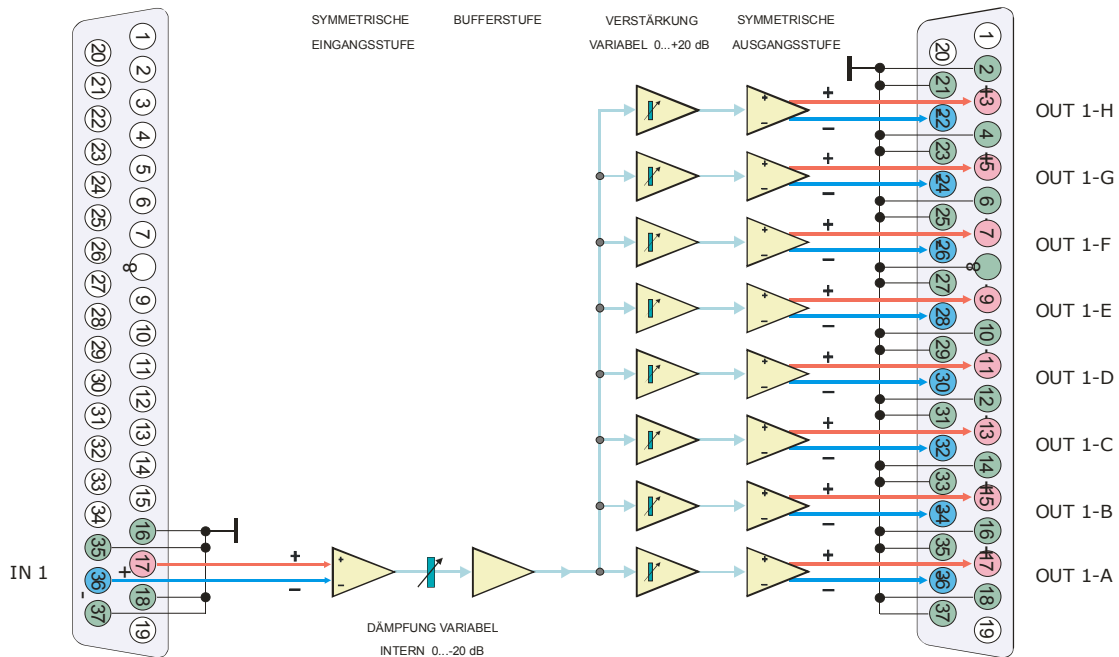
vollsymmetrischer Verteilverstärker SAM-3B.V2/8v1
