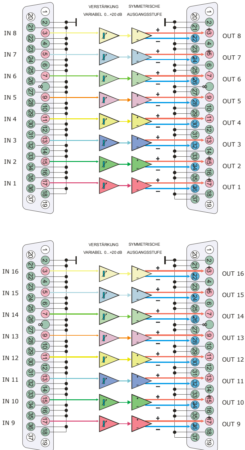
Symmetrierverstärker SAM-3B.V2/16-0
