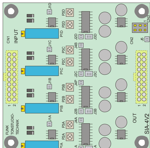
Lage der Jumper und Steckverbinder
