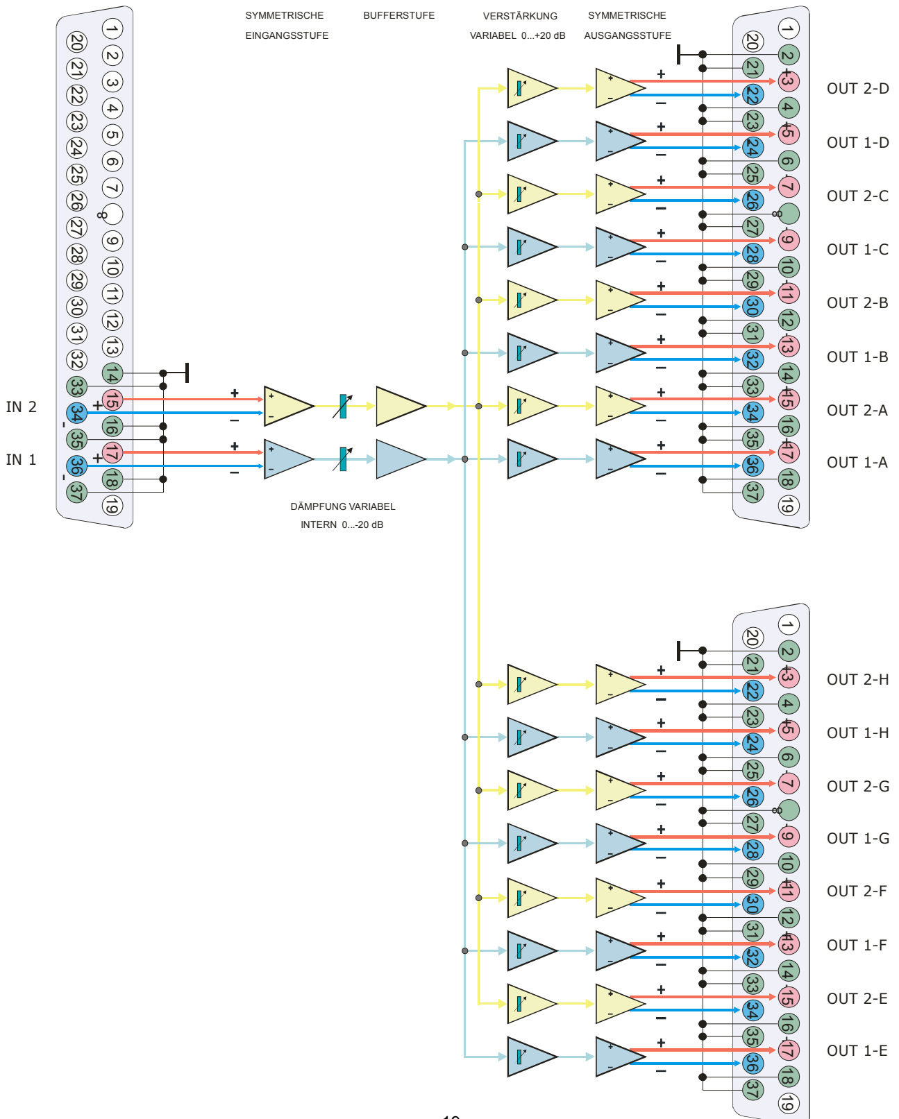
vollsymmetrischer Verteilverstärker SAM-3B.V2/16v2
