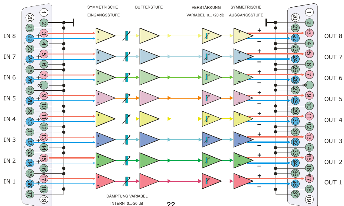
vollsymmetrischer Anpassverstärker SAM-3B.V2/8SVS8
