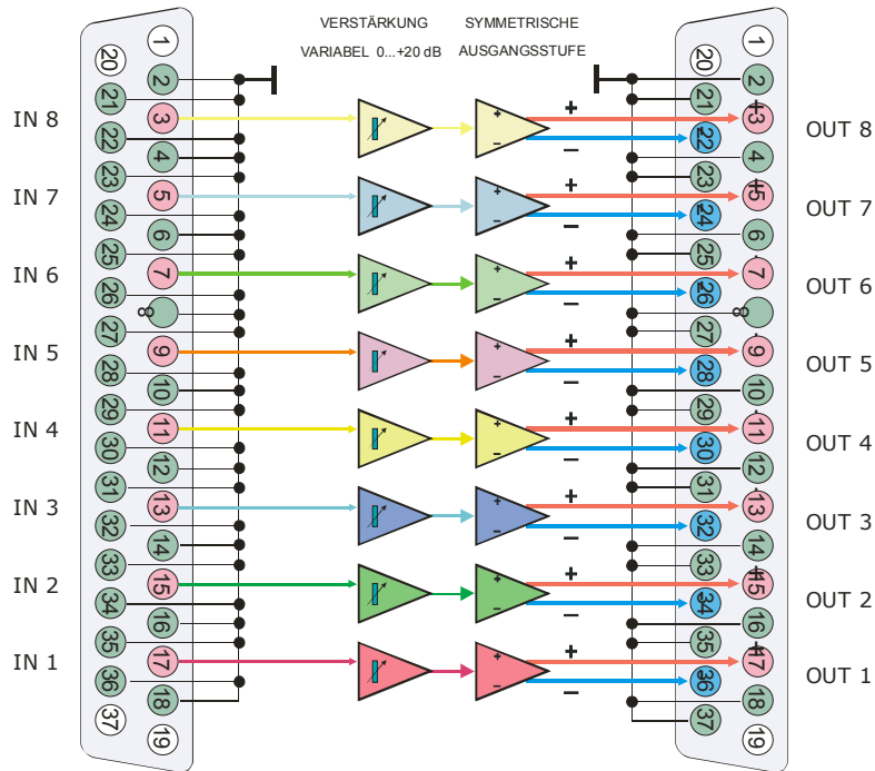
Symmetrierverstärker SAM-3B.V2/8-0
