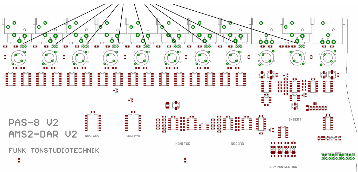
Jumper für Eingangsimpedanz
