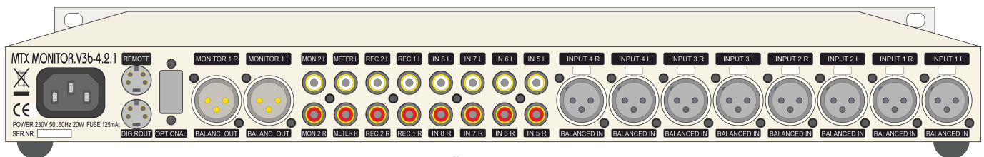
RÜCKWAND
