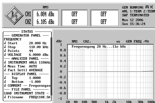
Frequenzgang Monitorweg 20 Hz...110 kHz Skala : +/- 1dB
