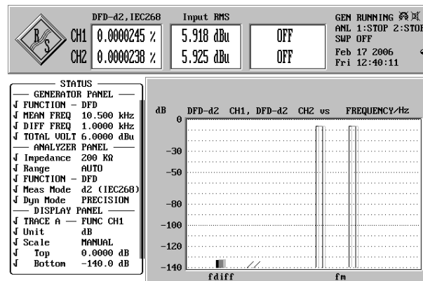
Differenzfrequenz-Verzerrungen bei +6 dBu Leitungspegel
