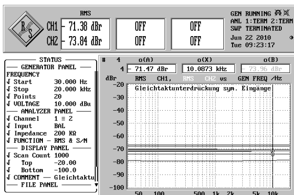
Gleichtaktunterdrückung aller sym. Eingänge über Frequenz
