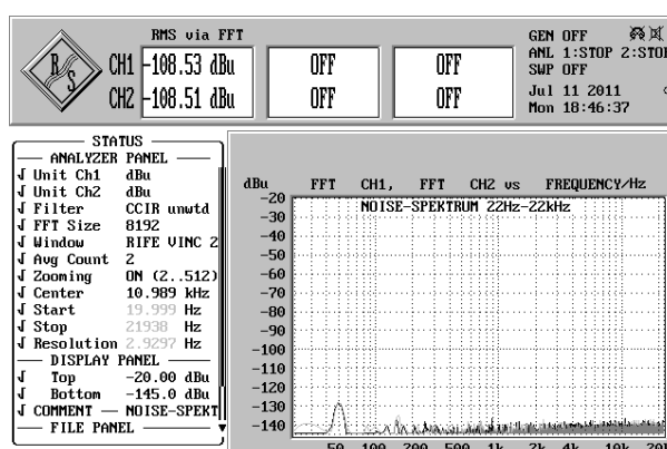
„Noise“-Spektrum Recordausgang (Cinch)
