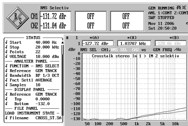
Übersprechen Eing. 1 L+R auf Eing. 2 (mit 47 \Omega abgeschlossen)
