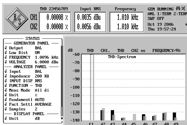
THD bei 1 kHz sym. Eingang > Record Out (k2..k9 bewertet)
